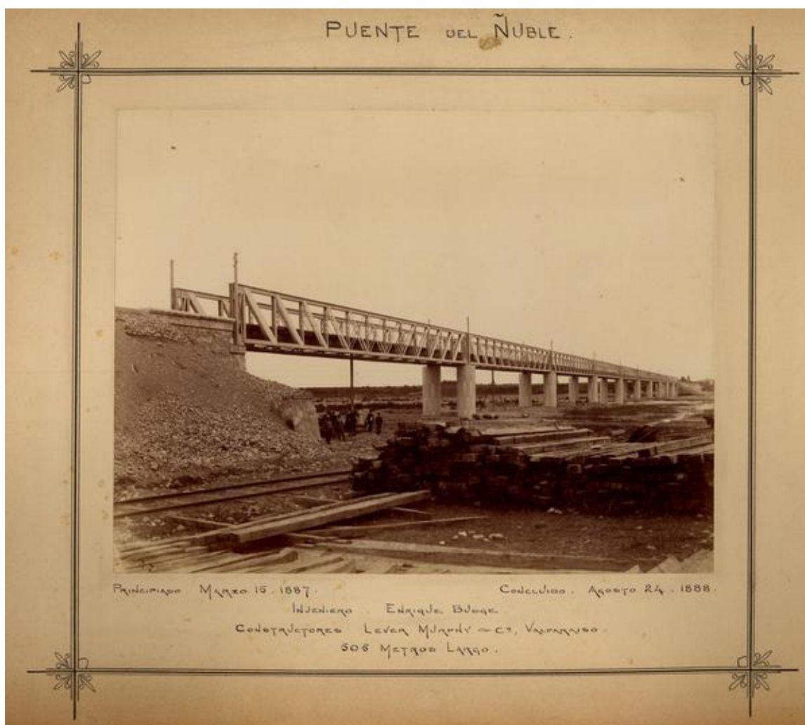
Puente del Ñuble: Puente del Ñuble: Principiado Marzo 15 1887-Concluido Agosto 24 1888-Ingeniero Enrique Budge-Constructores Lever Murphy & Ca., Valparaíso. 505 Metros Largo. [fotografía].
