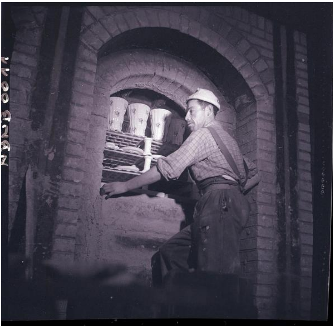
[Horno de producción de cerámica] [fotografía] Ignacio Hochhäusler.
