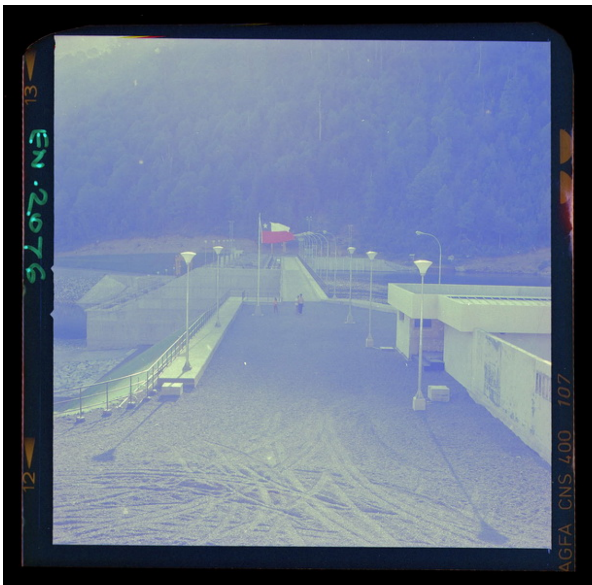
[Barrera móvil de la bocatoma Polcura] : Inauguración de la Central Antuco, 22 de octubre de 1981 [fotografía] Luis Ladrón de Guevara.
