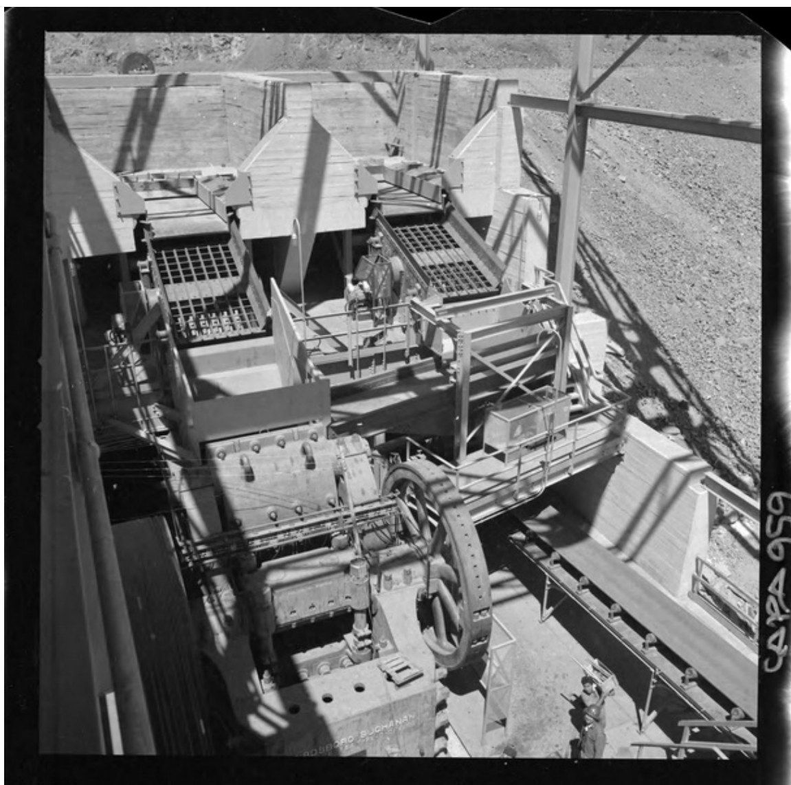
[Obras de construcción, equipo de minería Birdsboro-Buchanan; mina "El Algarrobo"] [fotografía] Luis Ladrón de Guevara.
