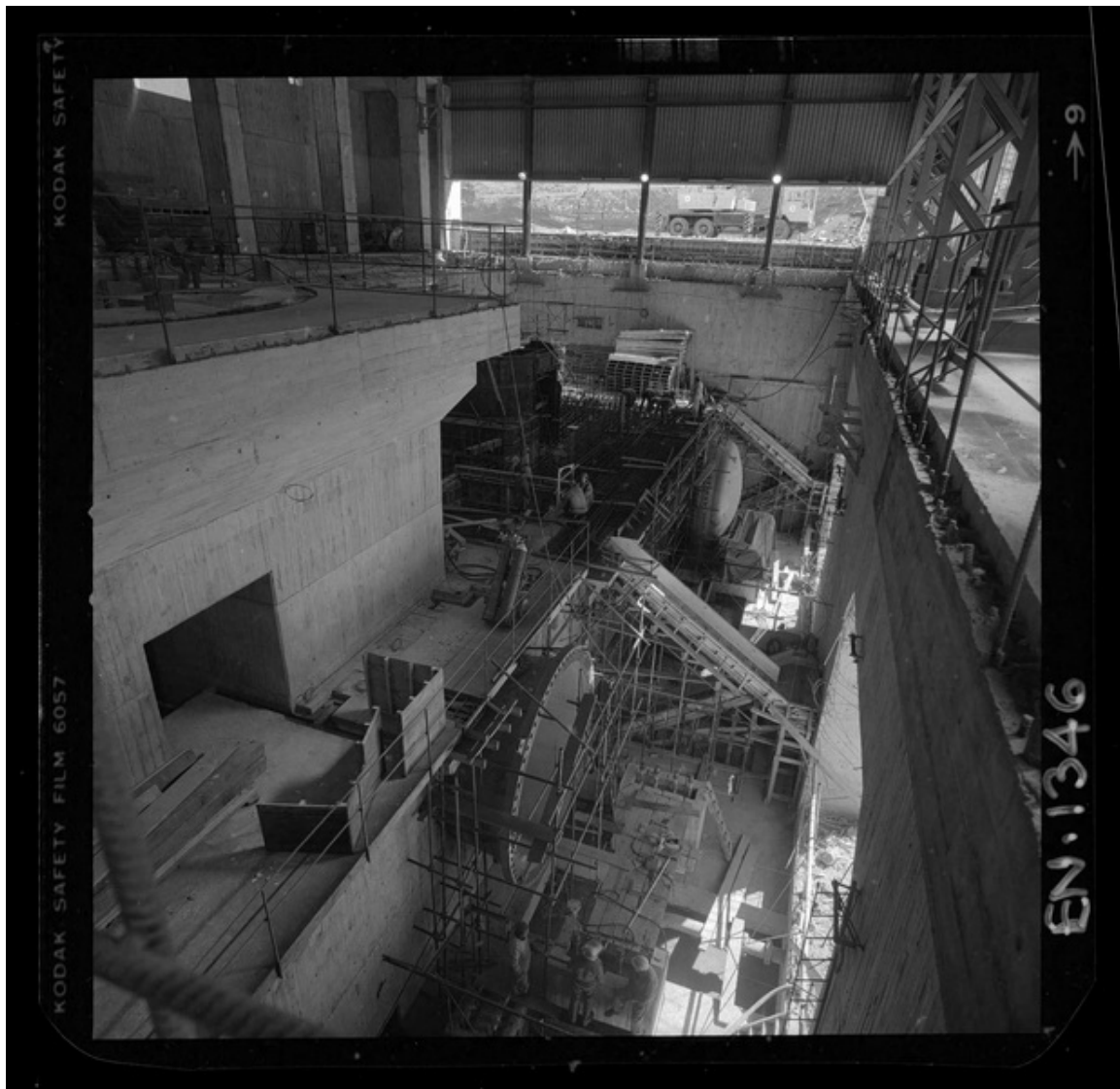
Casa de máquinas en una segunda etapa : vista exterior, interior y aspectos del montaje de los equipos, incluyendo el caracol de la turbina [fotografía] Luis Ladrón de Guevara.
