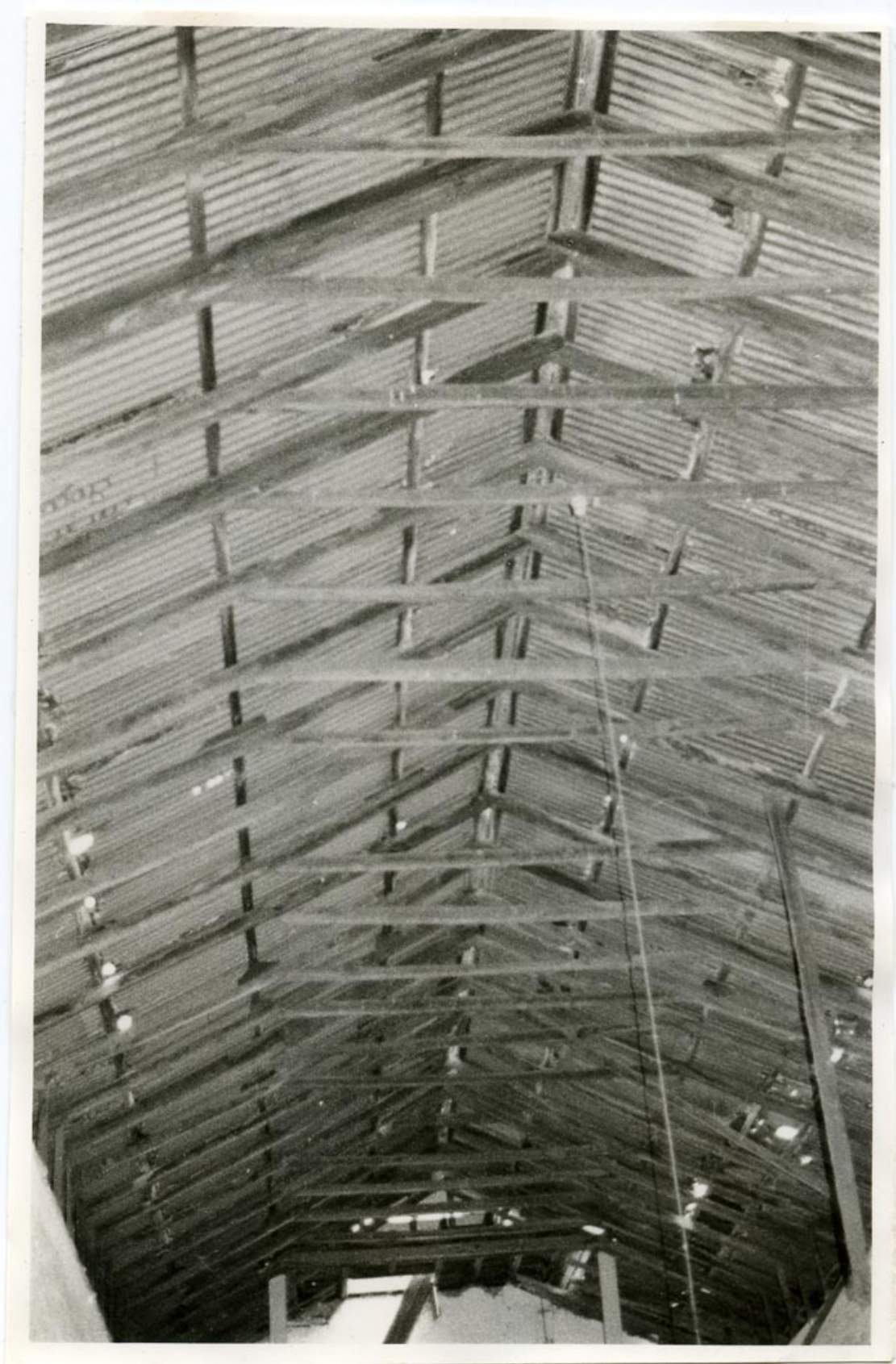
Detalle constructivo
