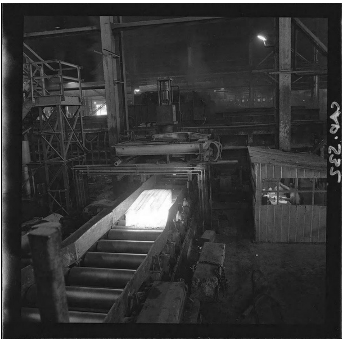
[Compañía de Acero del Pacífico : Alto Horno, fundición de acero Huachipato; proceso de laminación] [fotografía] Luis Ladrón de Guevara.
