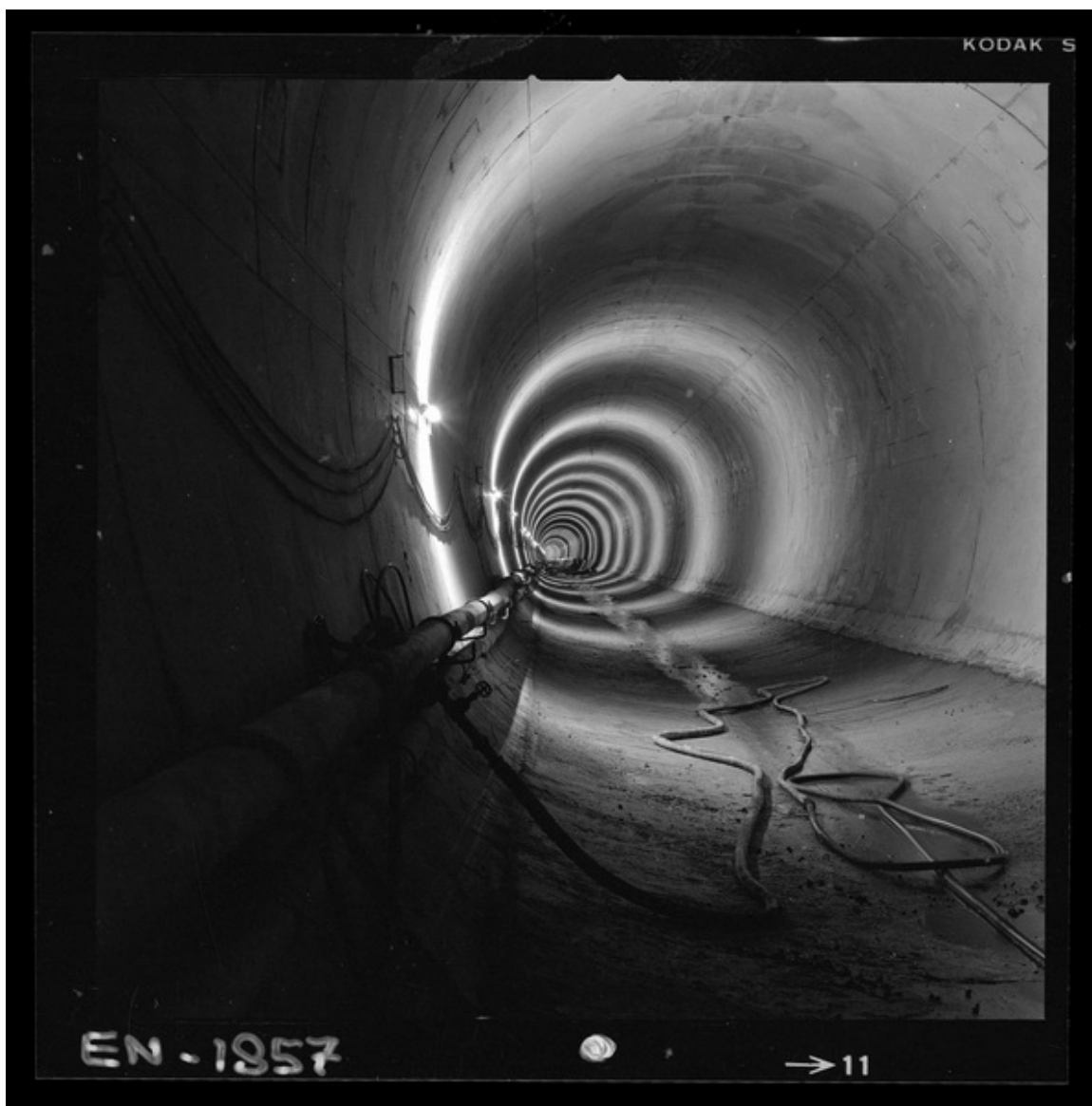
Aspecto de túneles en etapa de terminación, uso de moldajes retráctiles y hormigonado de bóveda [fotografía] Luis Ladrón de Guevara.
