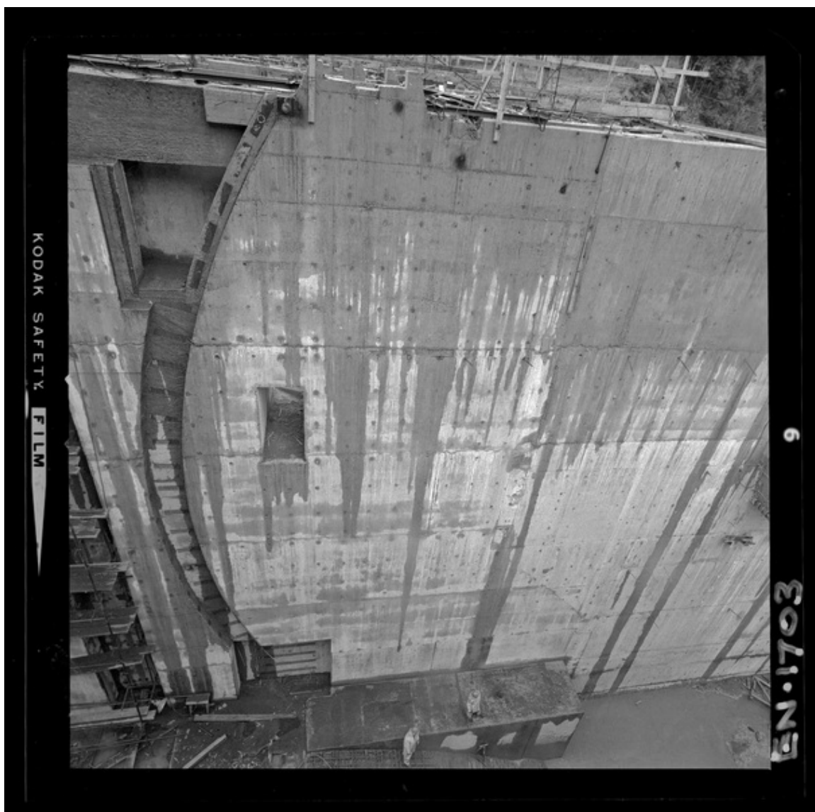
[Río Polcura; vista de las obras de construcción de la bocatoma Polcura] [fotografía] Luis Ladrón de Guevara.
